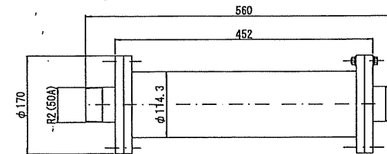
50A 重量 : 12Kg
