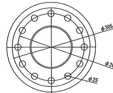
JIS20K圧カフランジ
