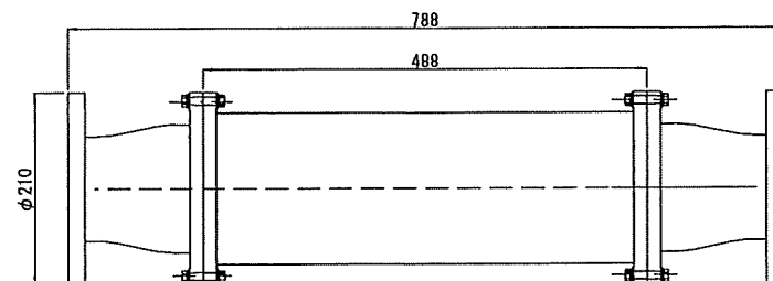
100A (10K) 重量 : 29Kg
