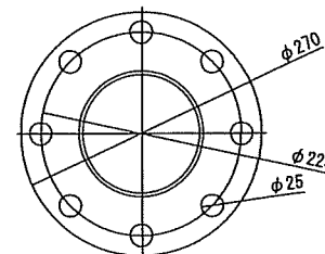
JIS20K圧カフランジ
