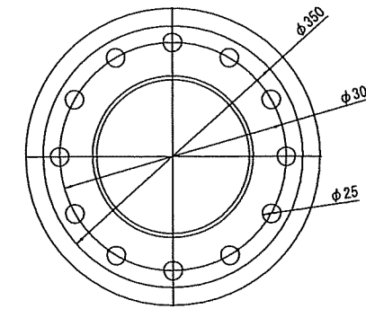
JIS20K圧カフランジ
