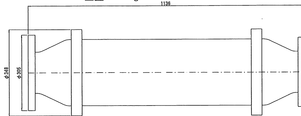
150A (20K) 重量 : 100Kg
