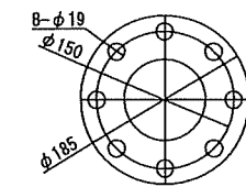
JIS10K圧カフランジ
