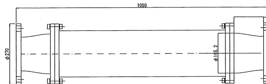
100A (10K) 重量 : 29Kg
