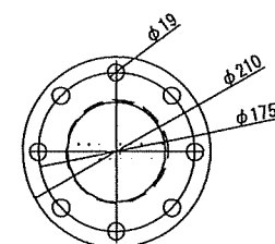
JIS10K圧カフランジ
